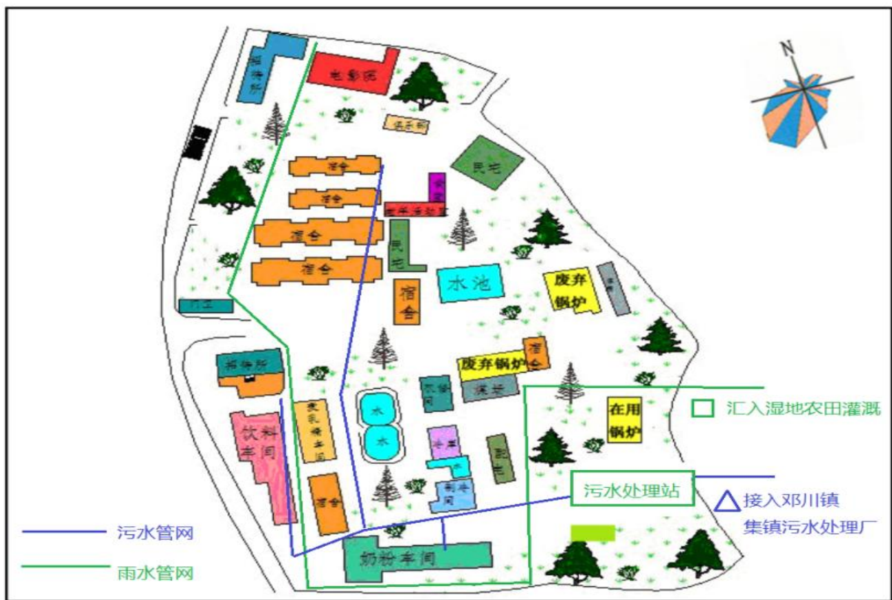
图2.1-2 云南新希望邓川蝶泉乳业有限公司老厂厂区总平面布置图
