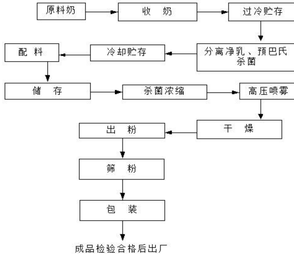
奶粉生产工艺流程图
